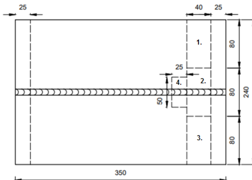
Slika 30. Zavarena ploča legure C-22, 350 \times 120 \times 6,35
