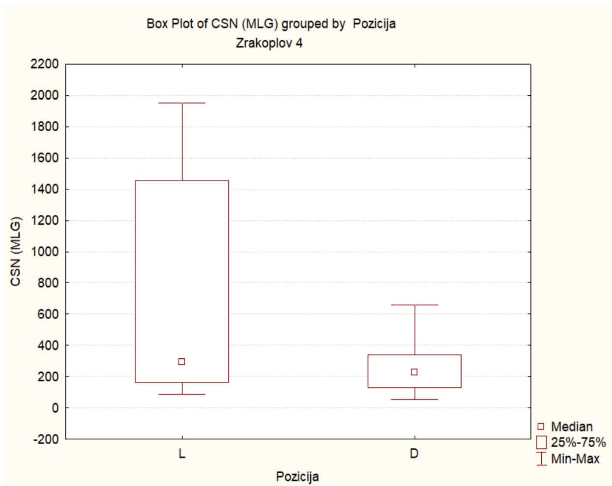
Slika 19. Usporedba varijabli broja slijetanja (CSN) za glavni stajni trap (MLG) između lijevog i desnog kotača Zrakoplova 4 (u donjem desnom kutu nalazi se legenda koja objašnjava značaj grafa)
