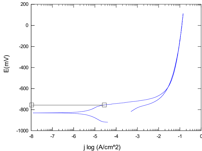
Slika 63. Ciklička polarizacija uzorka pri 40°C
