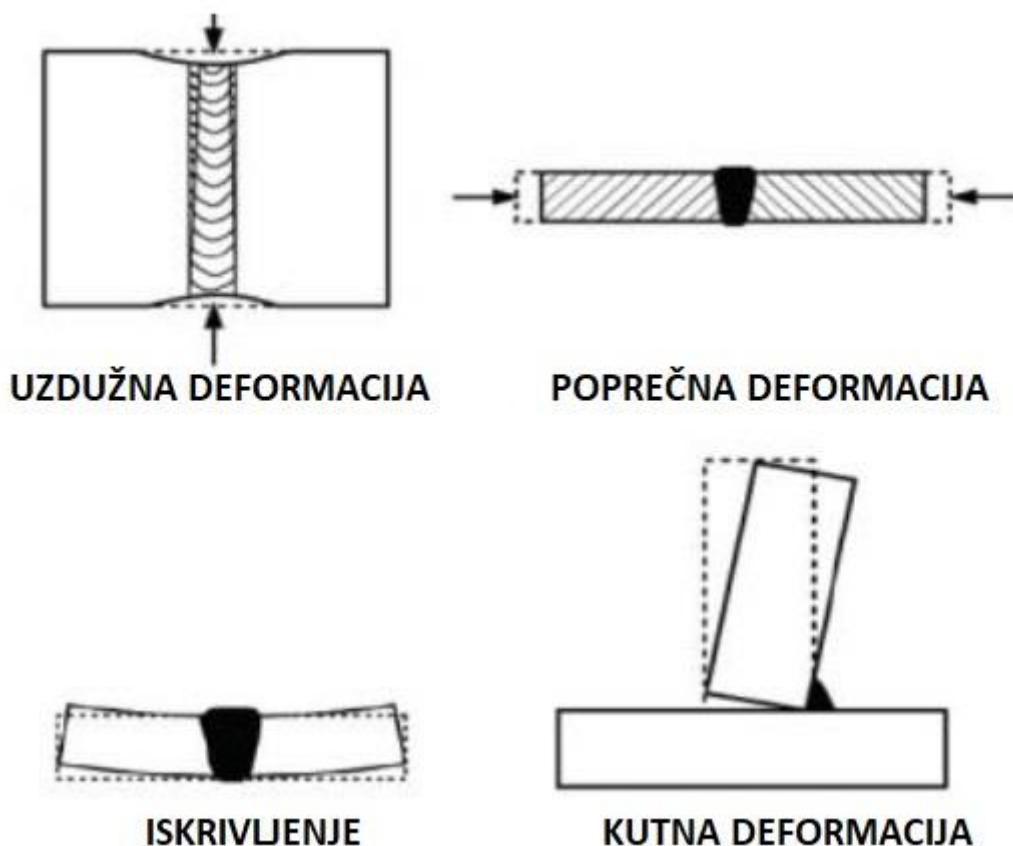
Slika 20. Vrste deformacija kod zavarivanja [30]
