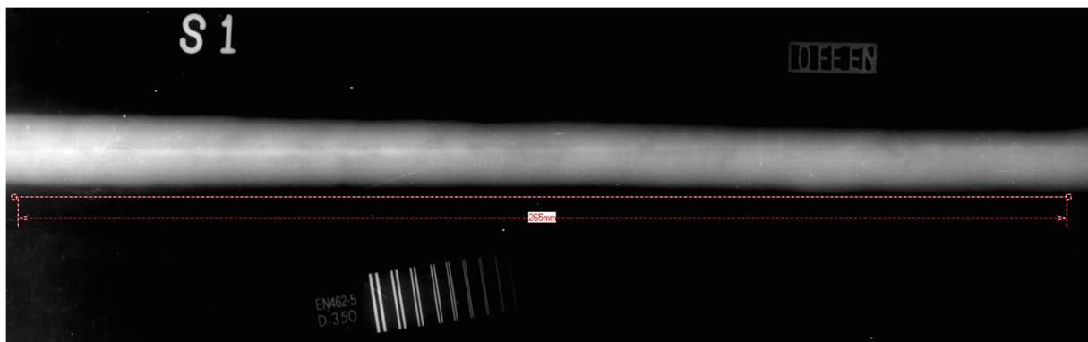
Slika 17. Radiogram ploče 1
