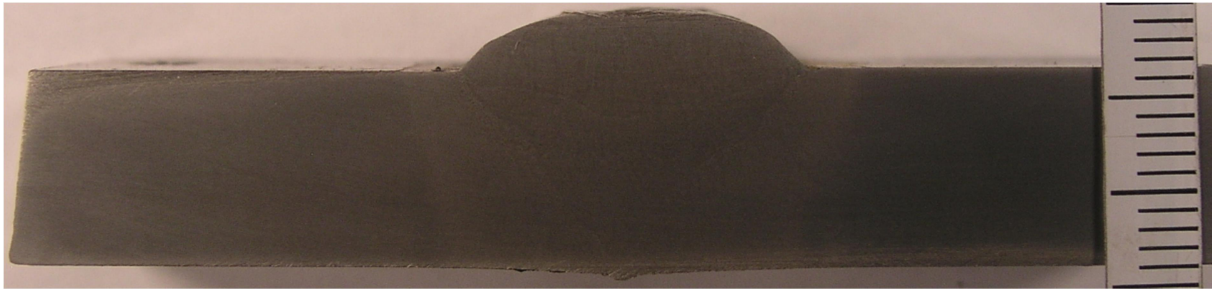
Slika 26. Makroizbrusak 1
