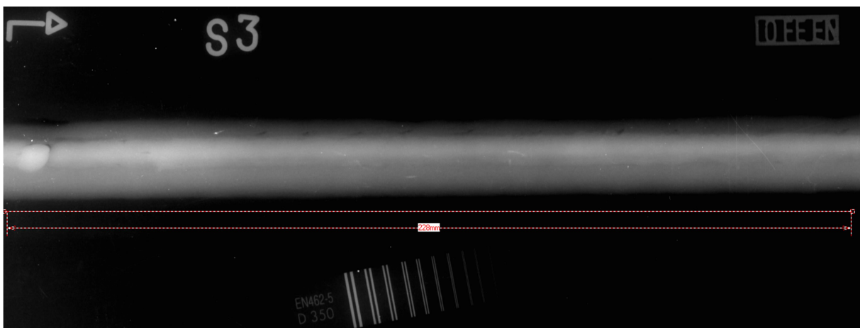
Slika 20. Radiogram ploče 3
