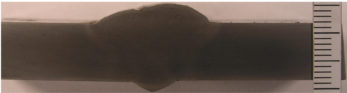
Slika 27. Makroizbrusak 2
