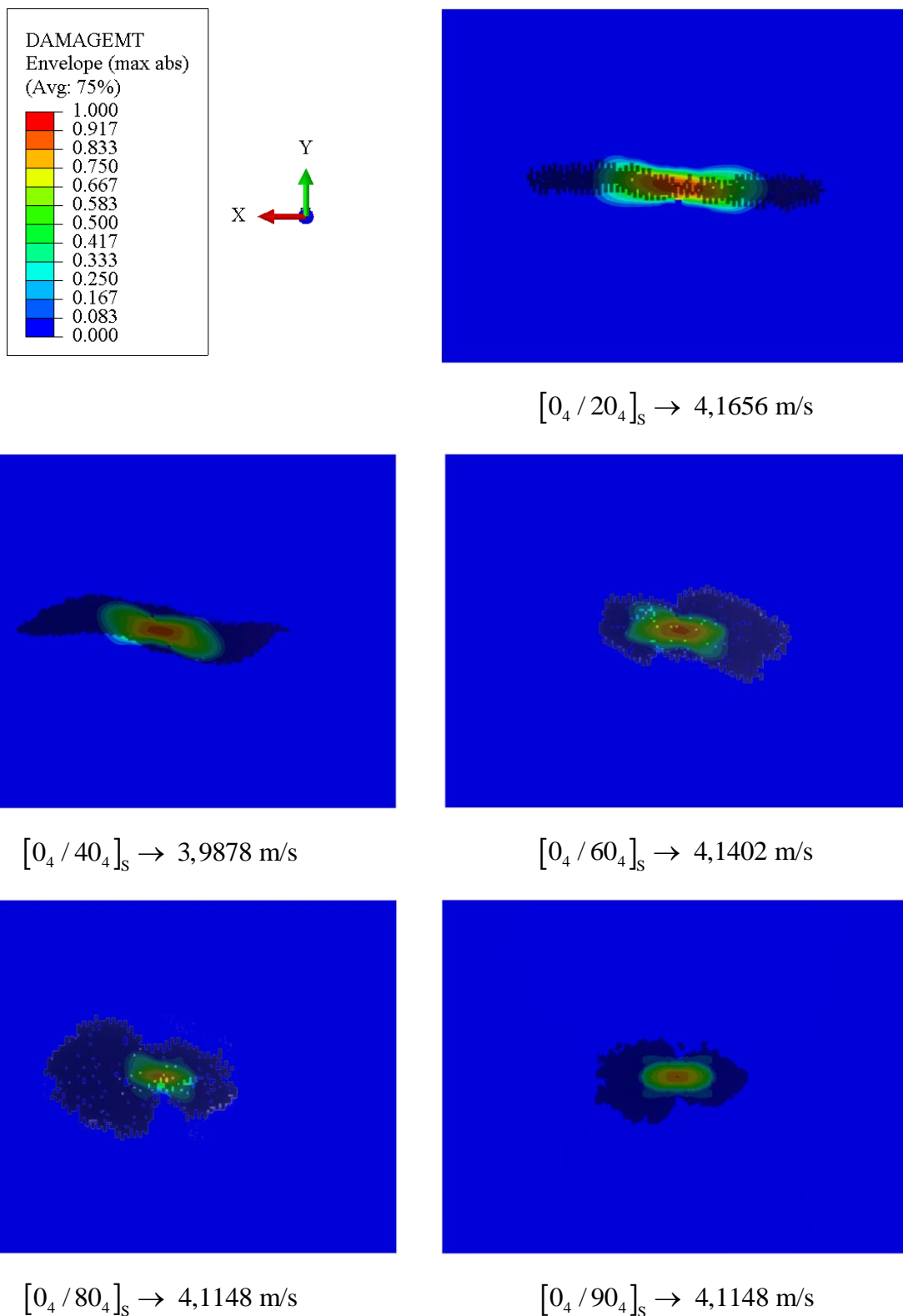
Slika 40. Prikaz rezultata DAMAGEMT varijable za modele različitih postavnih kutova korištenjem površina kohezivnog ponašanja
