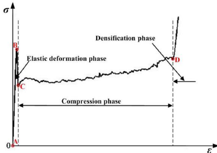
Slika 24: Stvarni materijalni model NOMEX-a [15]
