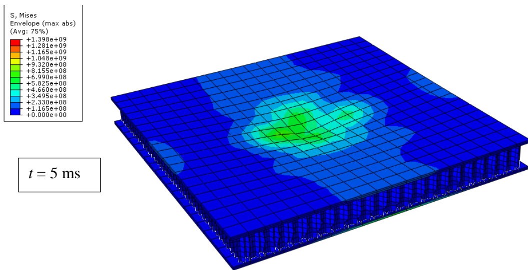
Slika 54: Raspodjela napreznja po Von Misesu [Pa] za sačasti model za energiju udara 10J i kut udara 0^\circ
