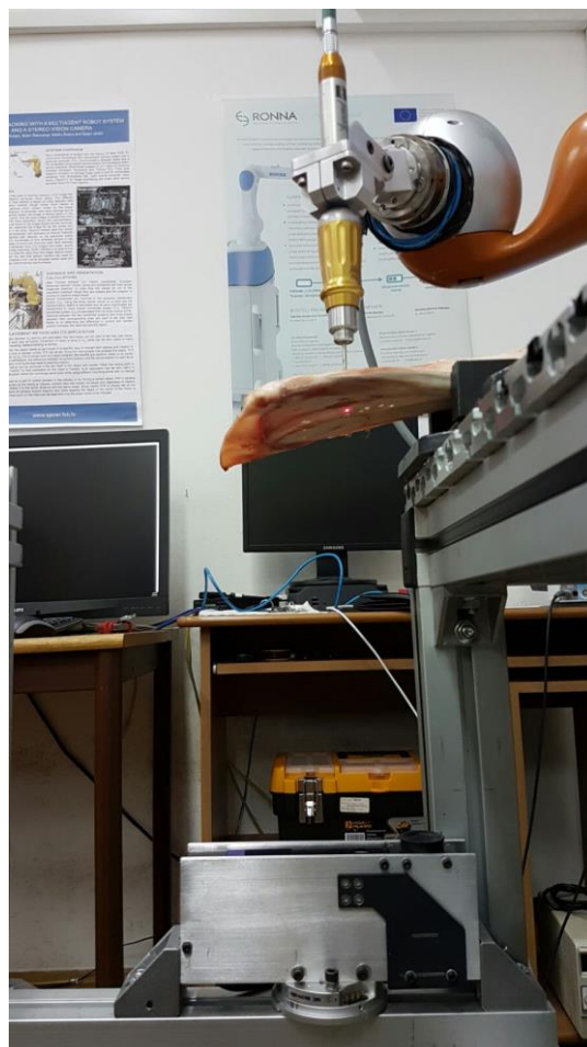
Slika 56. Kvantifikacija duljine hoda svrdla prilikom proboja
