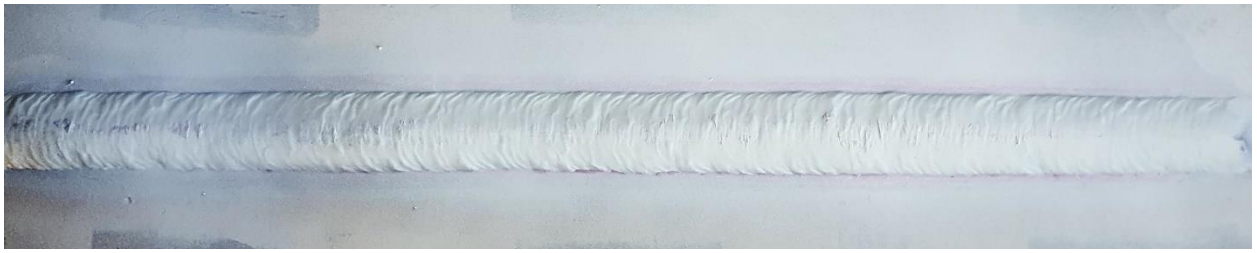
Slika 74. Uzorak A s nanesenim razvijačem - korijen zavara
