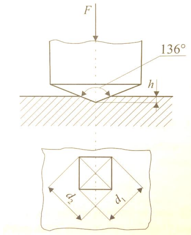
Slika 61. Skica penetratora i otiska kod Vickersove metode [24]
