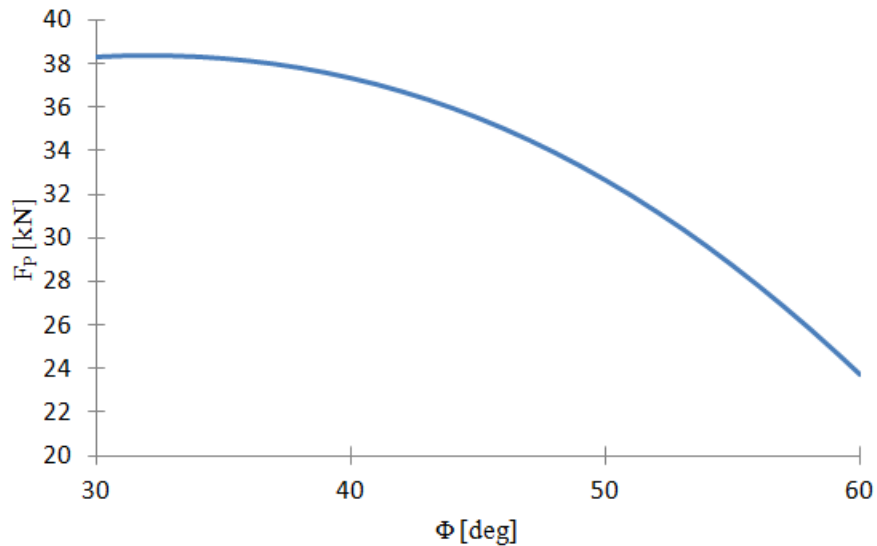
Slika 36. Dijagram ovisnosti poprečne sile u dohvatniku s obzirom na kut nagiba dohvatnika
