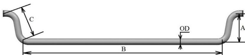
Slika 50. Pogled na prednji poprečni stabilizator sa dimenzijama koje su u skladu sa ranije definiranimima
