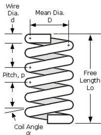
Slika 30. Dimenzije opruge
