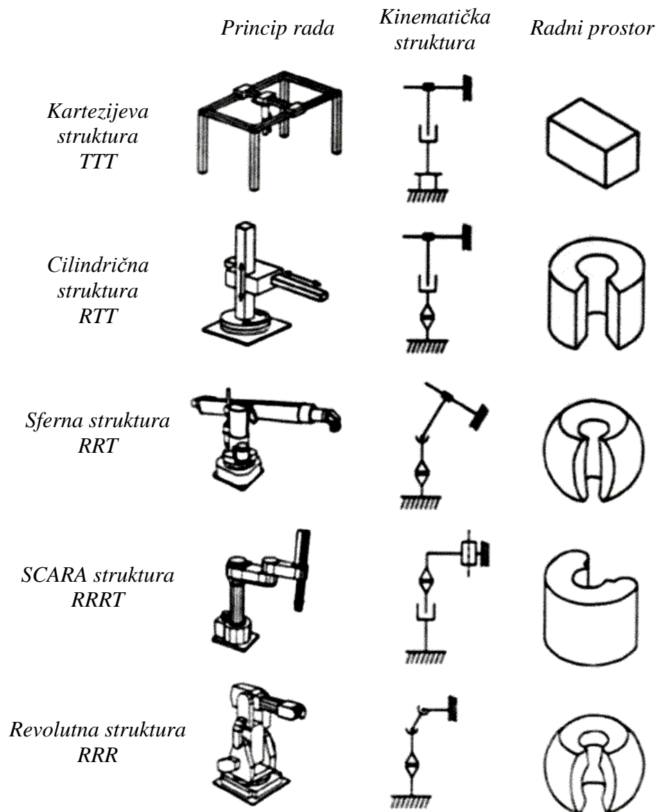
Slika 2. Strukture komercijalnih industrijskih robota
