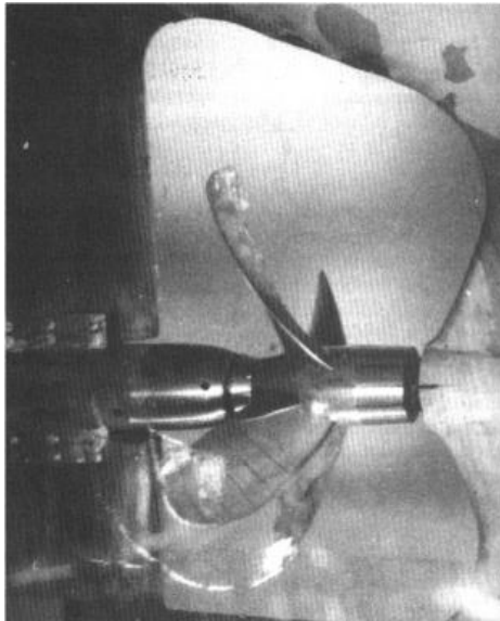
Slika 16. Mjehurićasta kavitacija [3]
