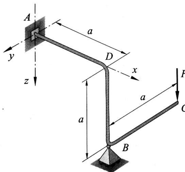
Slika 20. Prostorna gredna konstrukcija [7]
