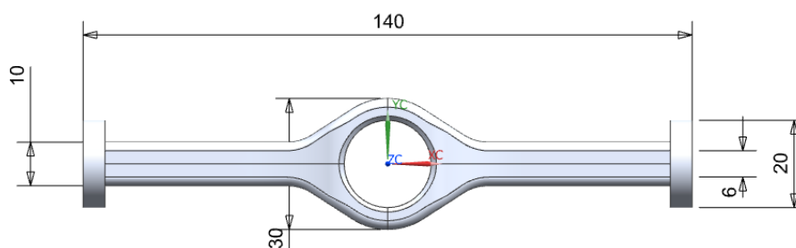
Slika 6. Dimenzije kućišta
