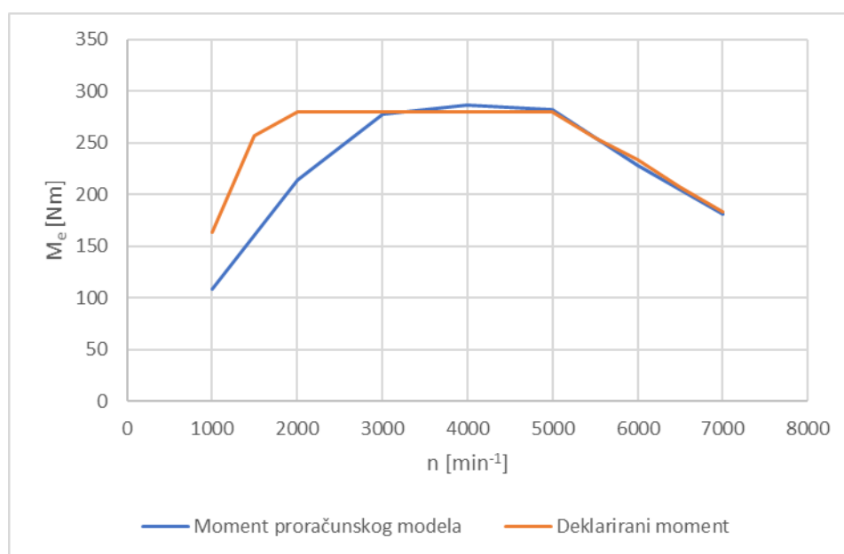
Slika 17. Usporedba momenta proračunskog modela i deklariranog momenta
