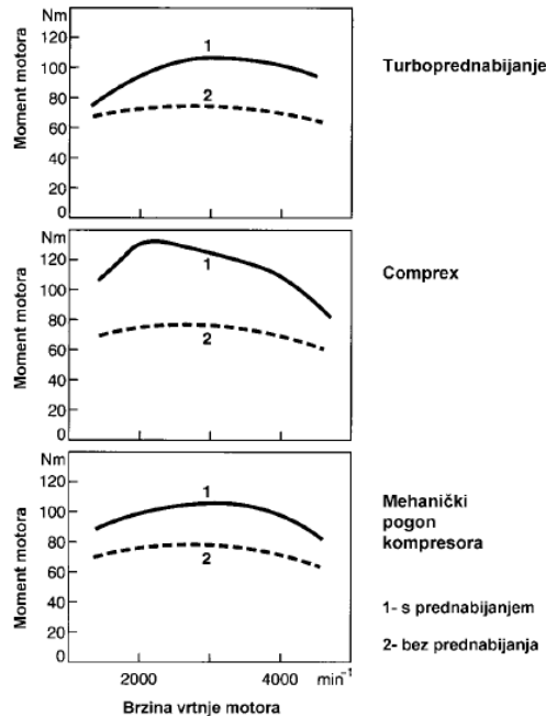
Slika 3. Usporedba motora sa i bez nabijanja pri različitim tipovima nabijanja [2]
