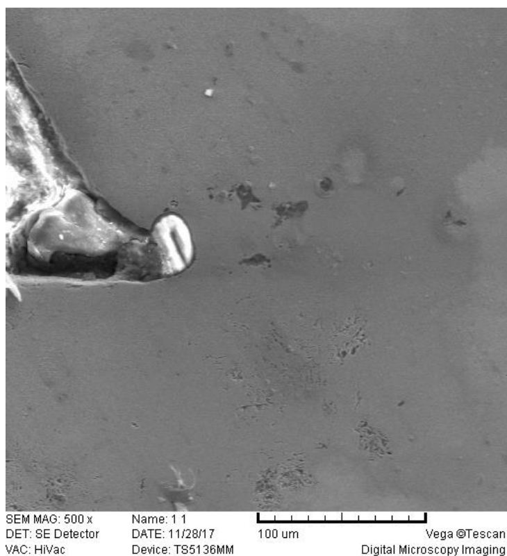
Slika 28. Segment šasije FIREWALL uzorak 1: detalj zavarava, SEM, porozitet
