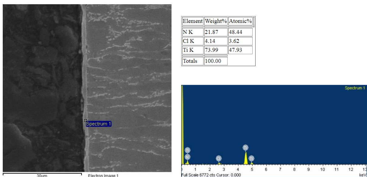
Slika 45. EDS analiza poprečnog presjeka uzorka prevučenog TiN prevlakom
