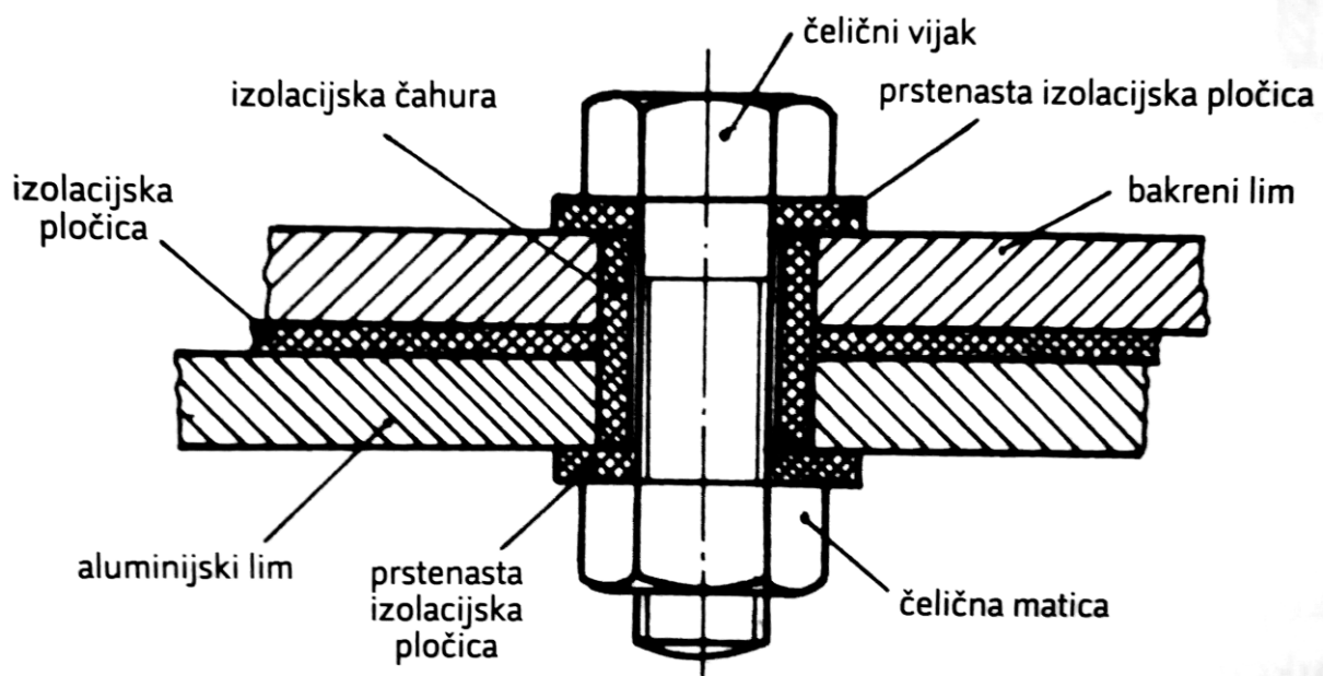
Slika 6. Vijčani spoj različitih metala s izolacijskim umecima [5]
