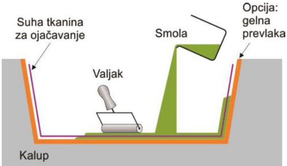
Slika 47. Postupak laminiranja – ručno polaganje [13]
