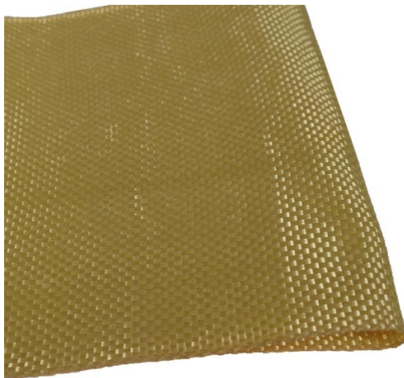
Slika 6. Aramidna vlakna [8]
