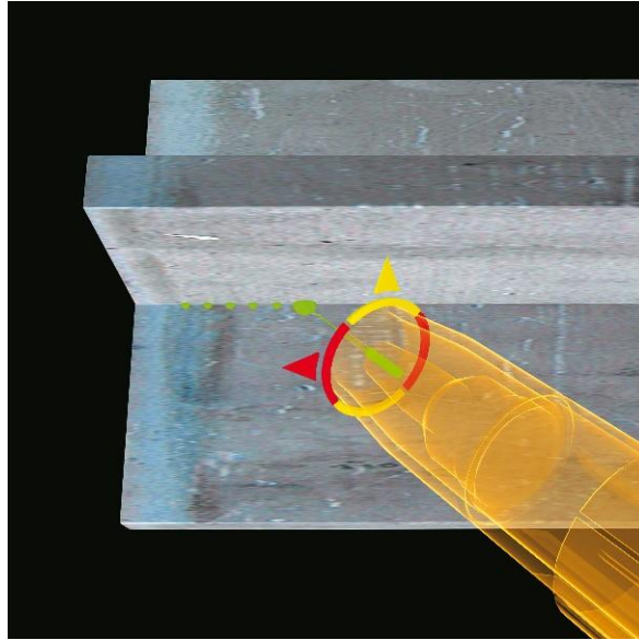
Slika 5. MIG/MAG simulacija [4]
