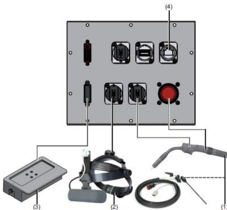
Slika 47. Priklučci opreme [6]
