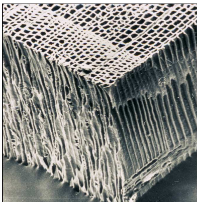
Slika 23. Celuloza
