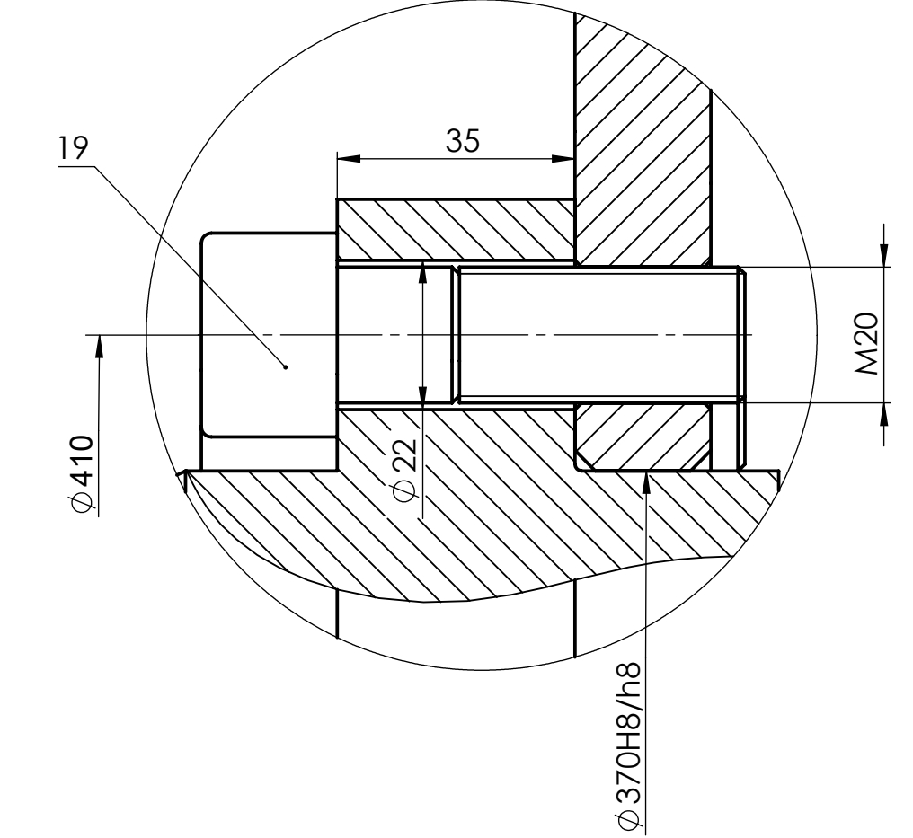
DETALJ D M 1:1
