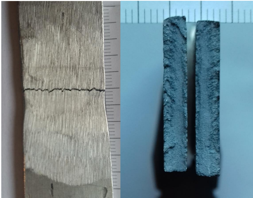
Slika 60. Epruveta 3-3
