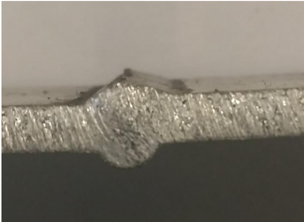
Slika 41. Epruveta prije brušenja
