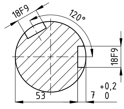
Presjek B-B M 1 : 2
