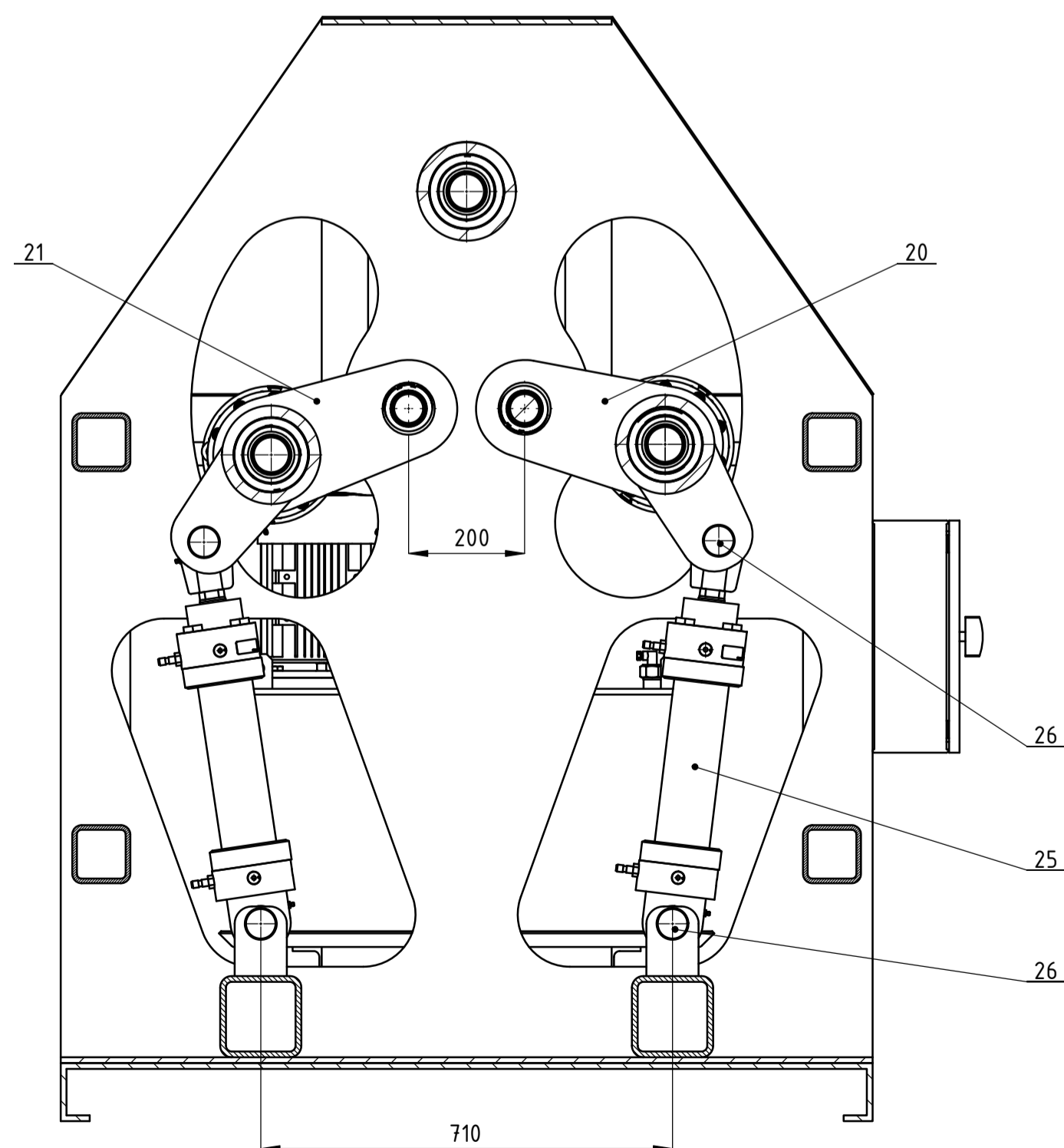
Presjek A-A M 1 : 10
