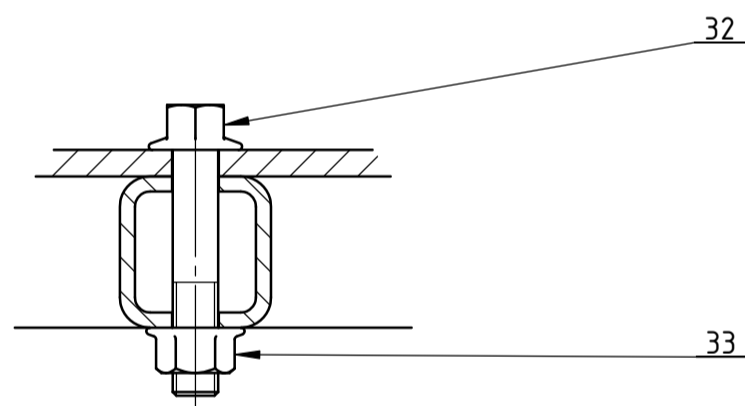
Detalj B M 1 : 2
