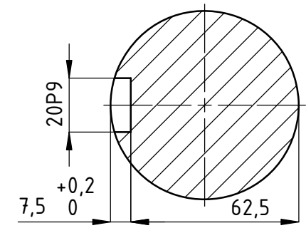
Presjek A-A M 1 : 2
