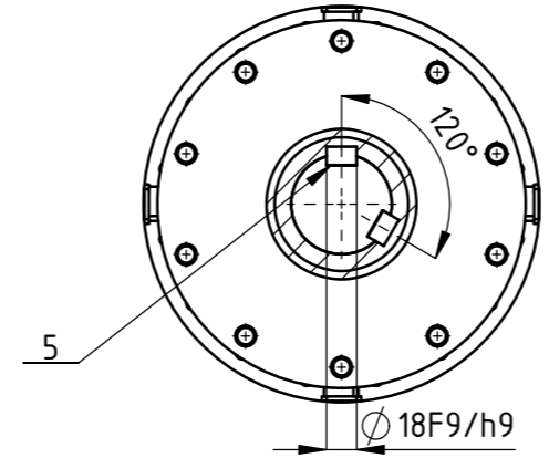
Presjek B-B M 1 : 5
