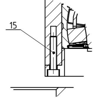
Detalj D M 1 : 2
