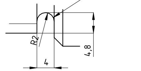
Detalj C M 2 : 1
