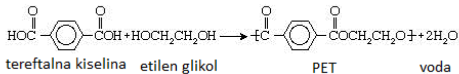
Slika 2.14. Formula PET-a [28]
