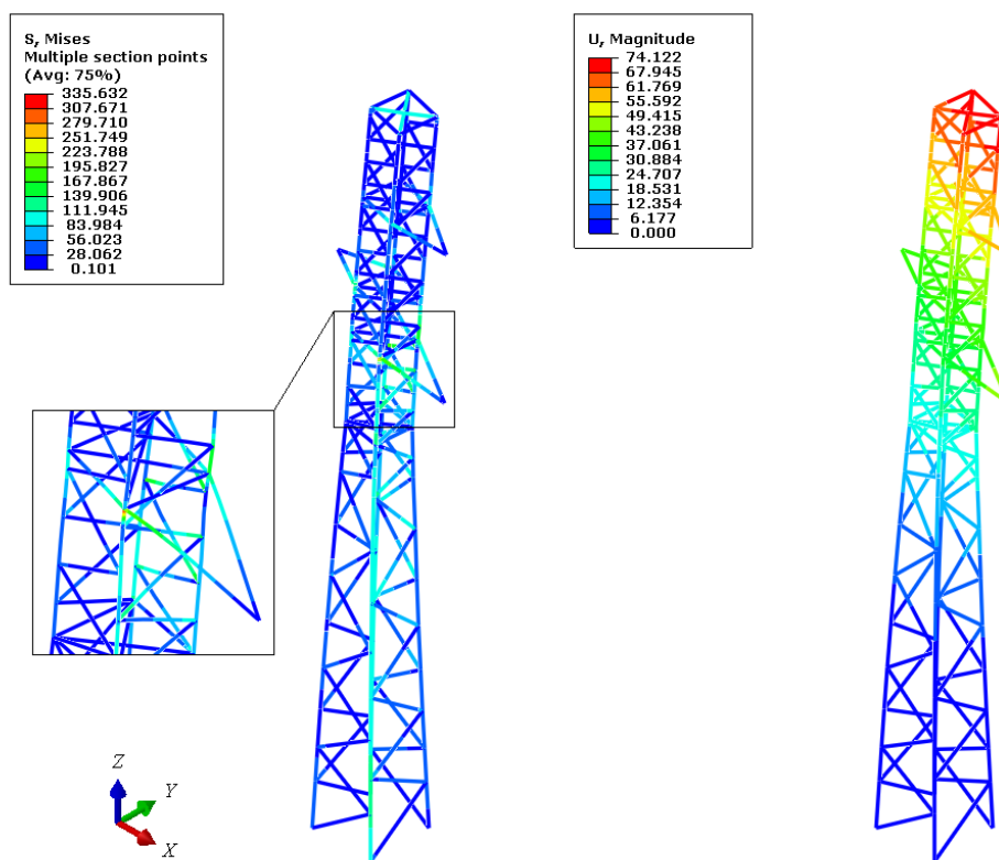
Slika 5.11. Raspodjela napreznaja (MPa) i pomaka (mm) za slučaj 69.2 P3
