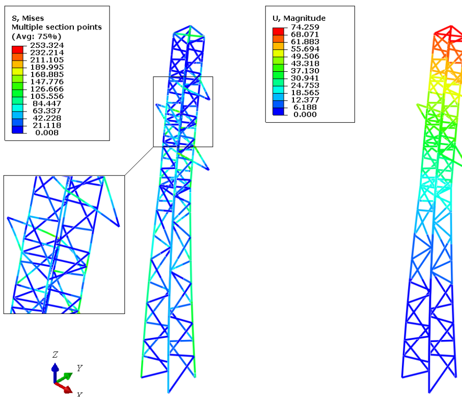
Slika 5.10. Raspodjela napreznanja (MPa) i pomaka (mm) za slučaj 69.2 P2
