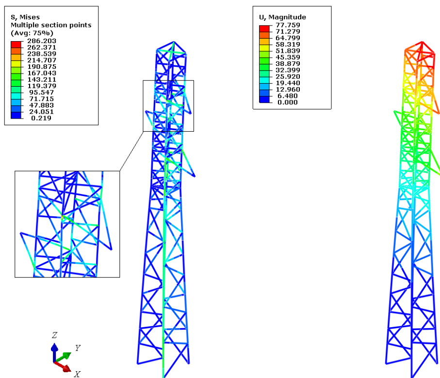
Slika 5.9. Raspodjela napreznanja (MPa) i pomaka (mm) za slučaj 69.2 P1
