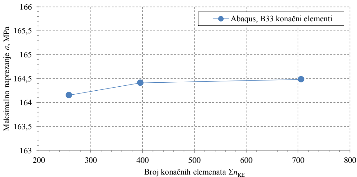
Slika 5.12. Dijagram ovisnosti maksimalnog napreznaja \sigma / MPa o broju KE
