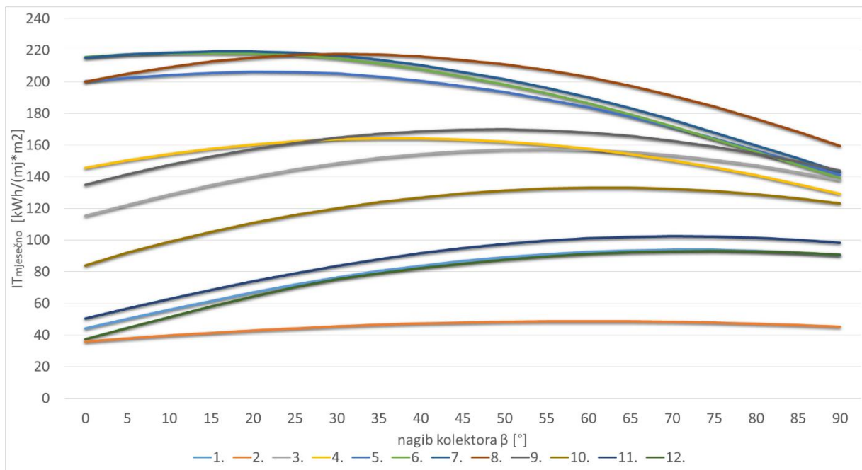
Slika 2.4. Mjesečno uprosječno sunčevo ozračenje u ovisnosti o nagibu kolektora
