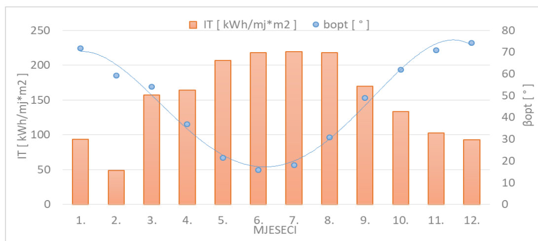
Slika 2.5. Maksimalno uprosječno sunčevo ozračenje uz optimalni nagib kolektora
