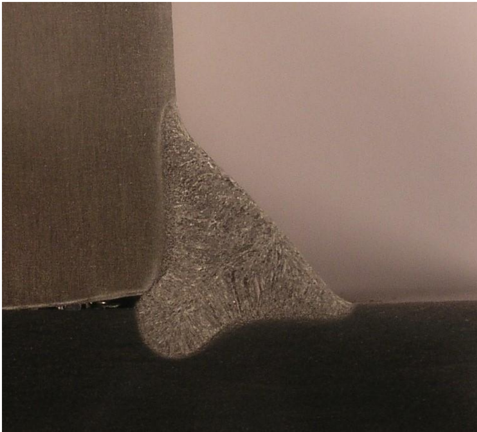
Slika 46 Makroizbrusak - uzorak 3
