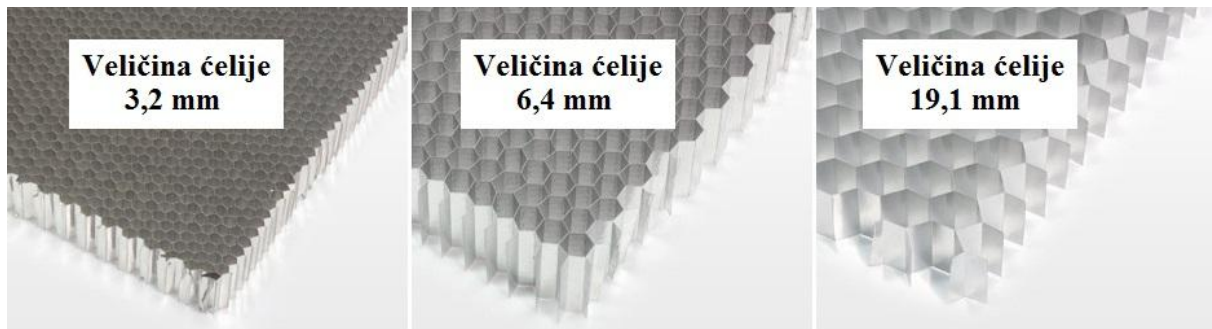
Slika 3.15. Aluminijske saće debljine h = 10 \text{ mm} [16]
