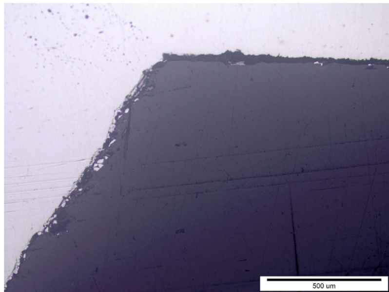
Slika 38. Oksidni sloj na korijenu zavora (pozicija 5)
