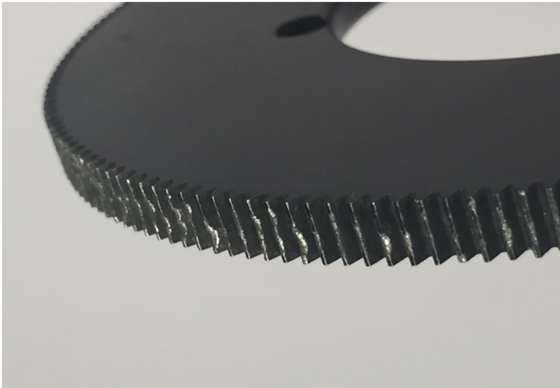
Slika 35. Makroskopska analiza tragoa trošenja velikog zupčanika
