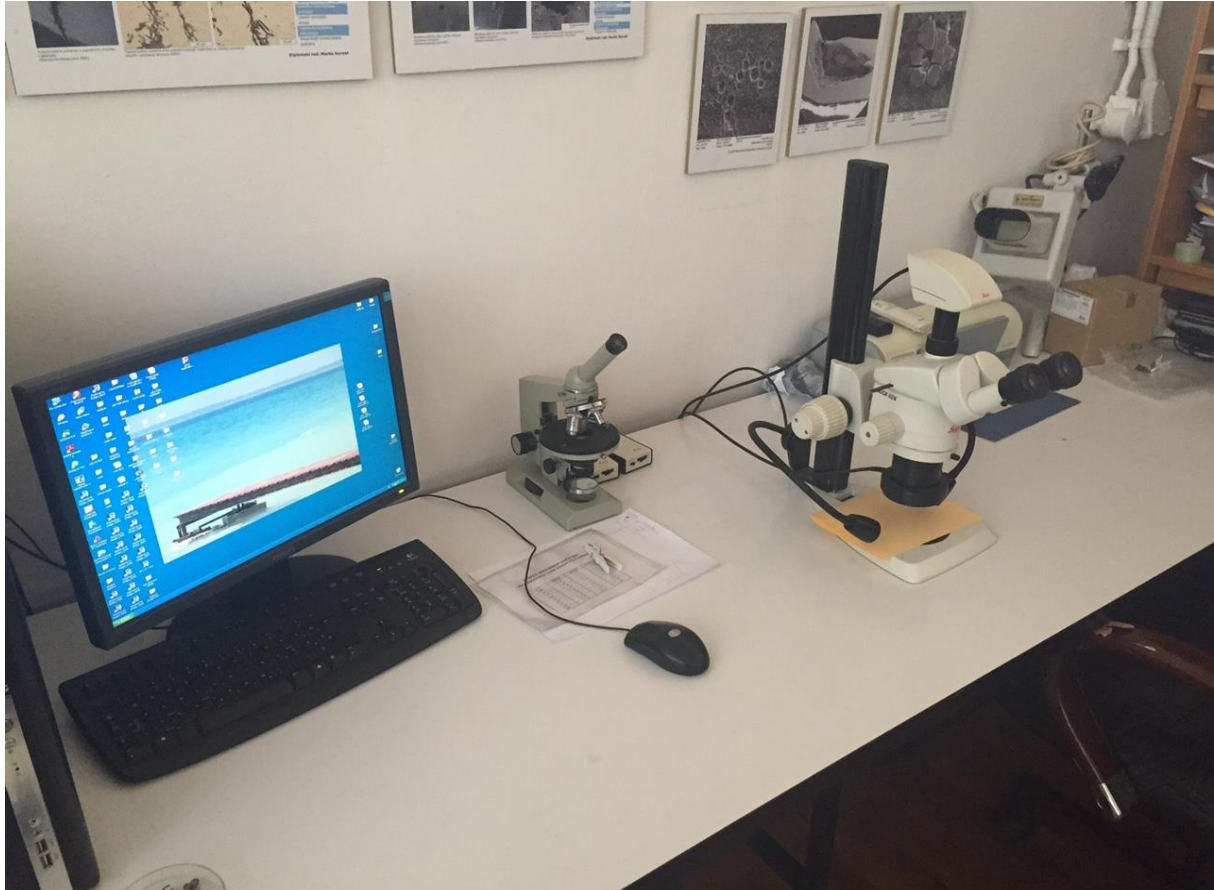
Slika 38. Stereomikroskopa Leica MZ6
