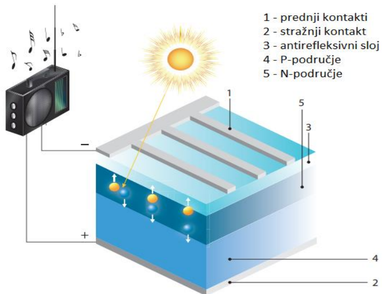
Slika 5. Fotonaponski članak [8]
