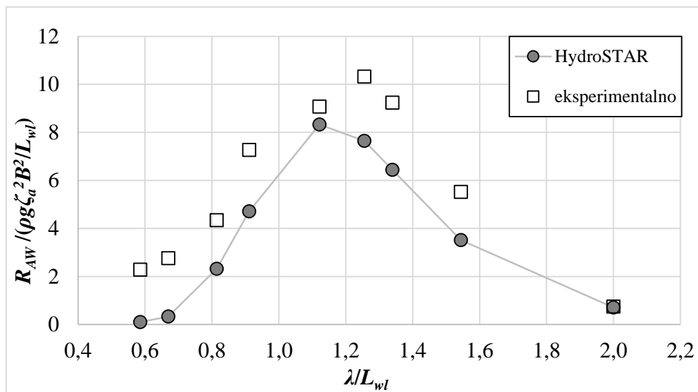
Slika 16. Usporedba numeričkih i eksperimentalnih rezultata za S175 pri Fr = 0,25
