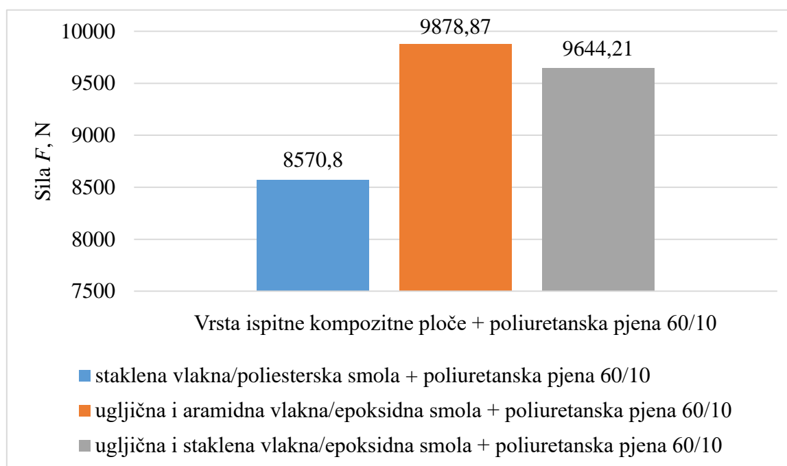
Slika 6.28. Usporedba rezultata sile F ispitnih na pločama s upotrebom poliuretanske pjene gustoće 60 \text{ kg/m}^3 i debljine 10 mm
