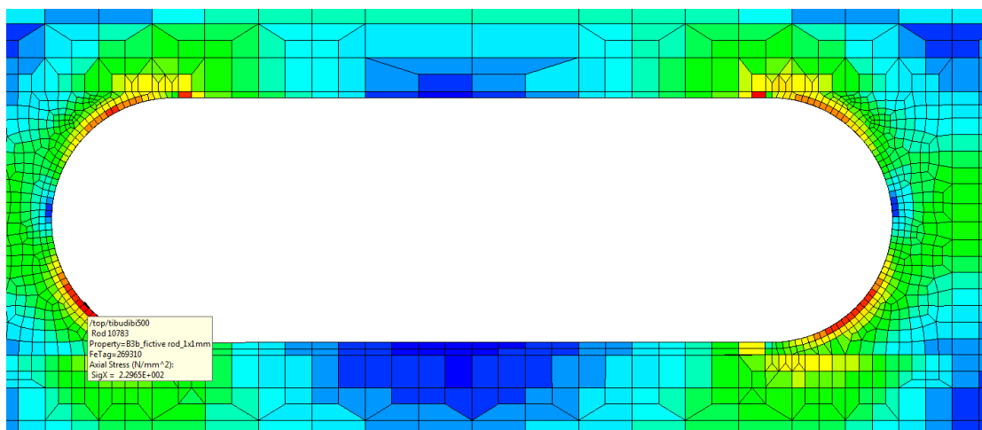
Slika 30. Očitavanje aksijalnog naprezanja sa štapnog elementa ( r = 500 mm)
