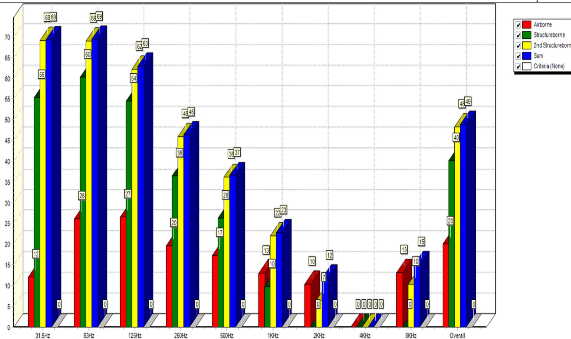
Slika 37. Razine buke za prostor kormilarnice (svi izvori buke aktivni, sa izolacijom)
