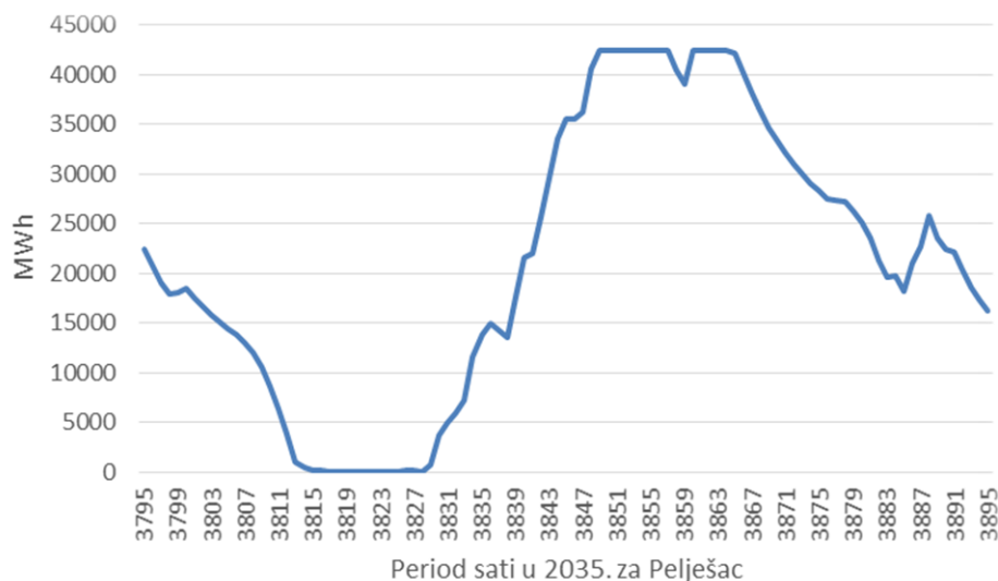
Slika 53 Kapacitet baterija. Pelješac 2035.
