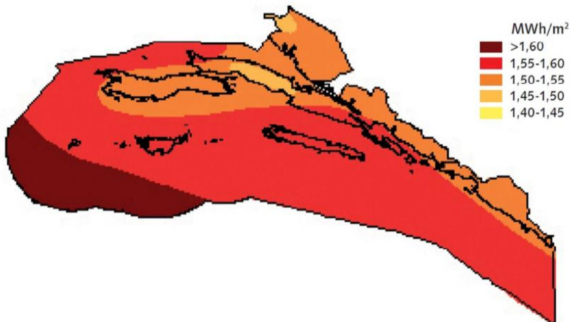
Slika 11 Srednja ozračenost vodoravne plohe na području Dalmatinsko-neretvanske županije (16)
