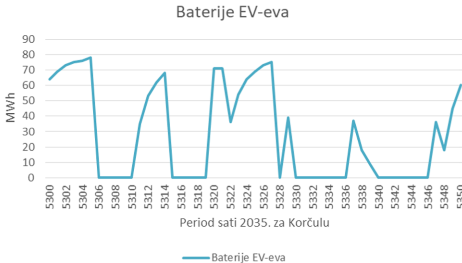
Slika 50 Kapaciteti baterije za period od 50 sati se koriste samo za pokrivanje transportnih potreba, Korčula 2035.
