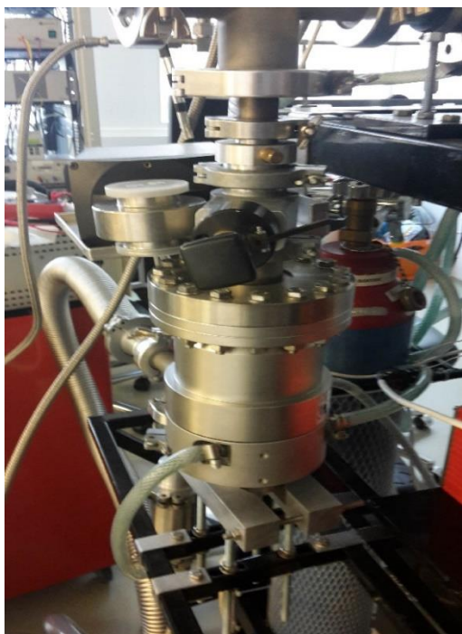
Slika 28. Turbomolekularna pumpa
