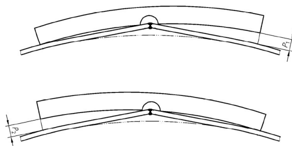
Slika 7: Mjerenje vanjskog izbočenja [11]
