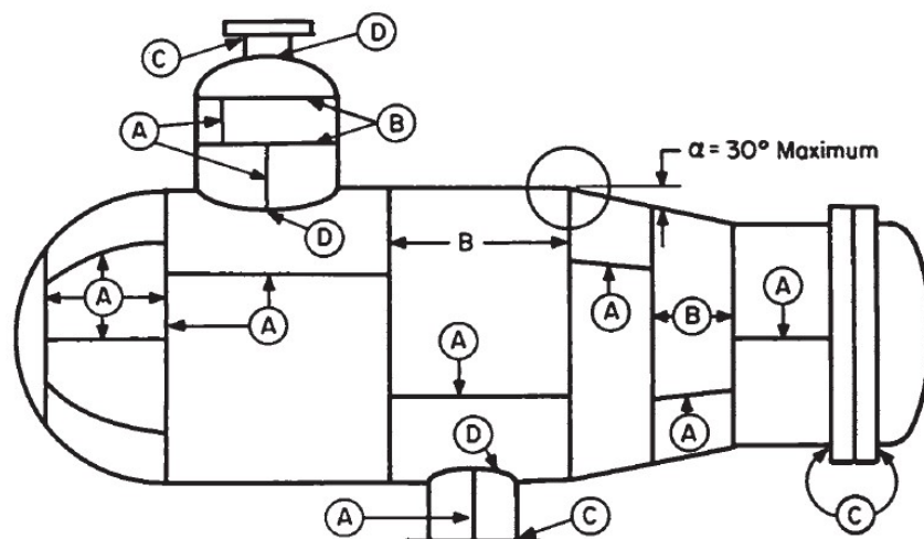
Slika 4: Kategorije zavarenih spojeva na posudu pod tlakom [10]
