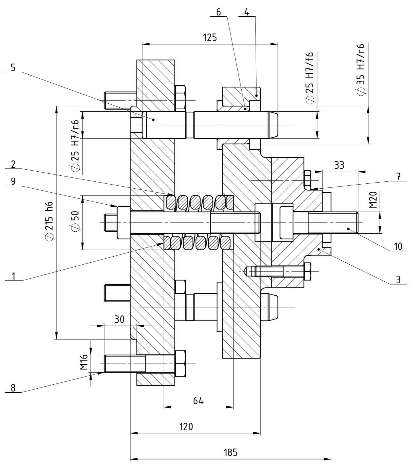
A-A (1 : 2)
