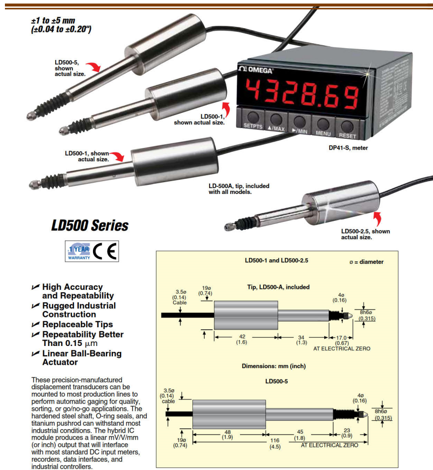
Slika 33. Senzor položaja [35]
