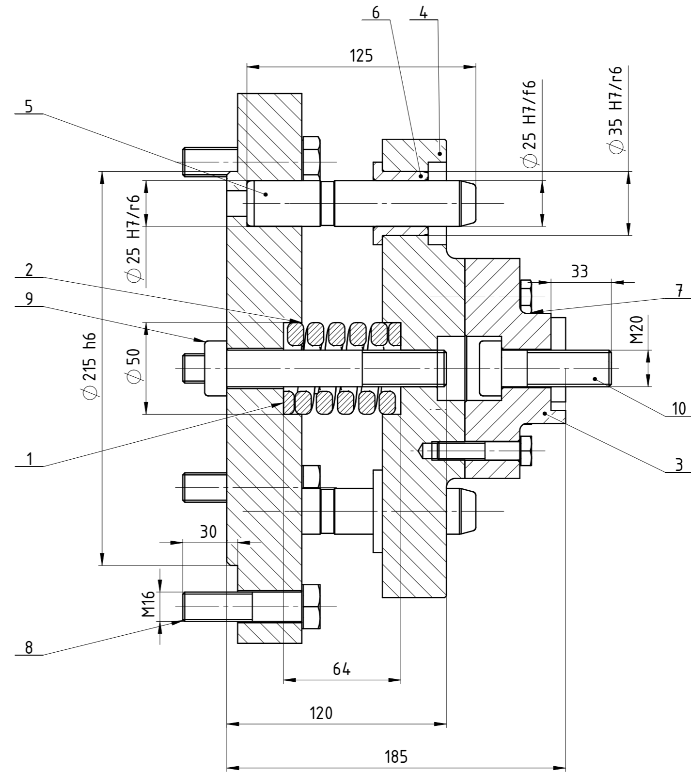
A-A (1 : 2)
