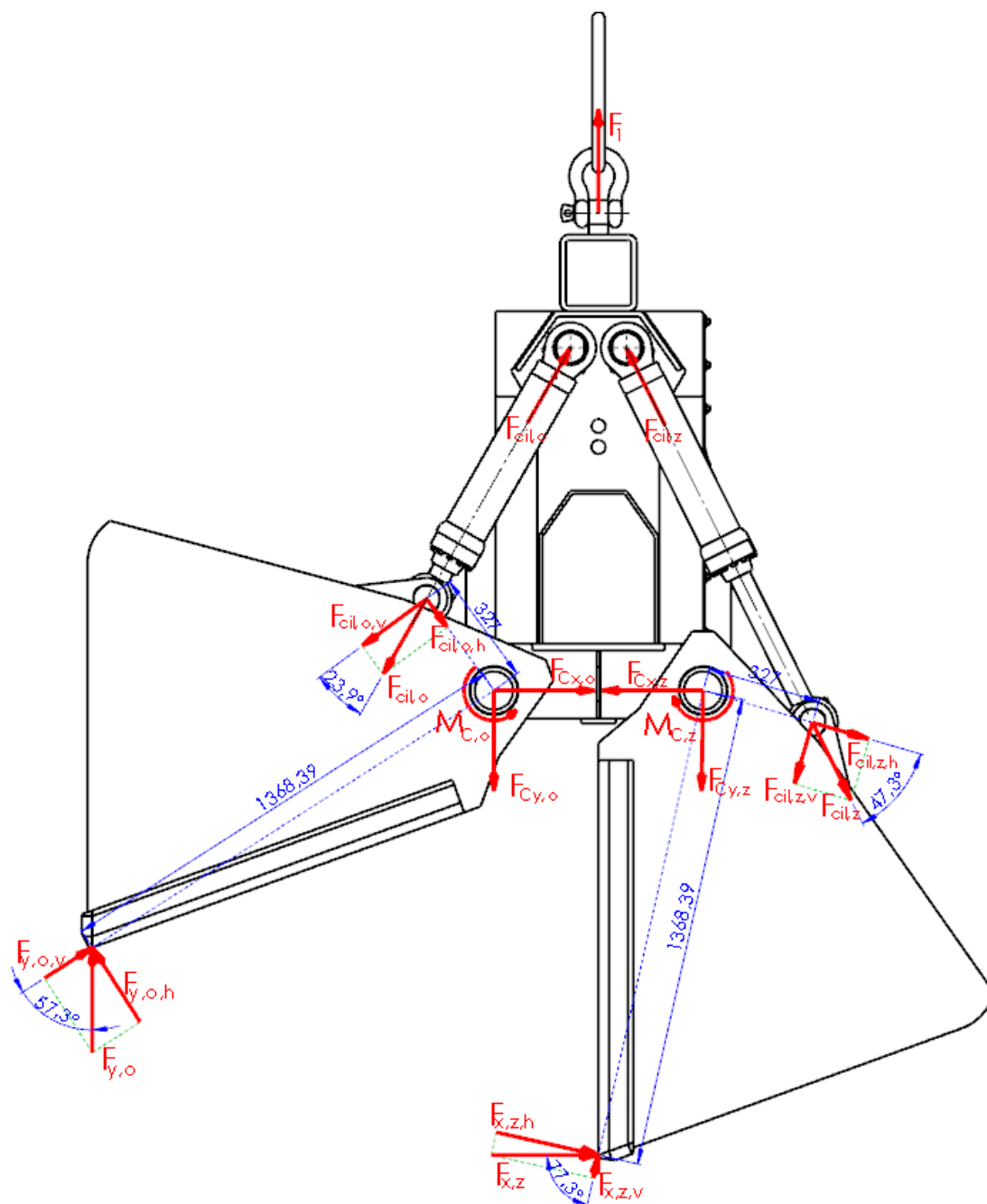
Slika 12. Sile koje djeluju na grabalicu potrebne za određivanje sile u cilindru
