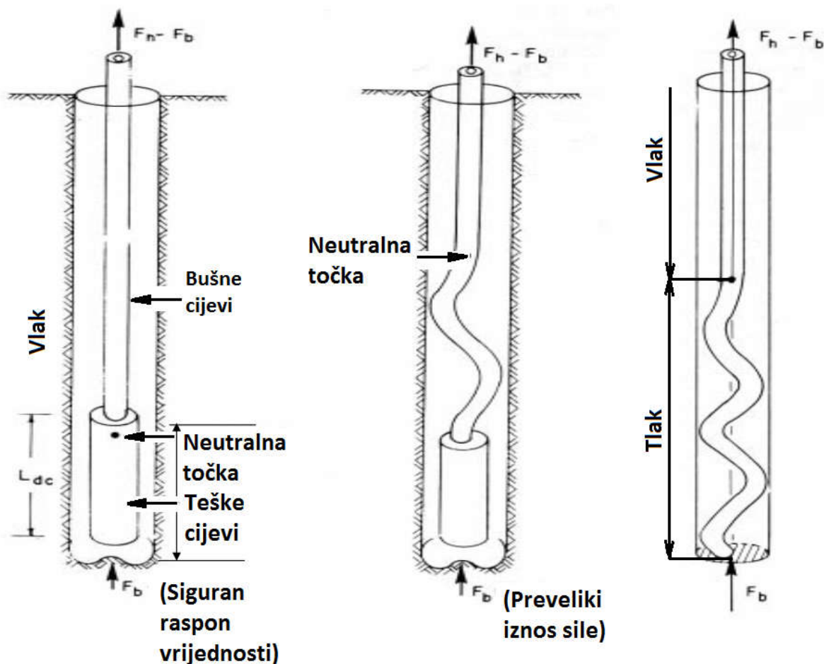
Slika 13 Izvijanje cijevi
