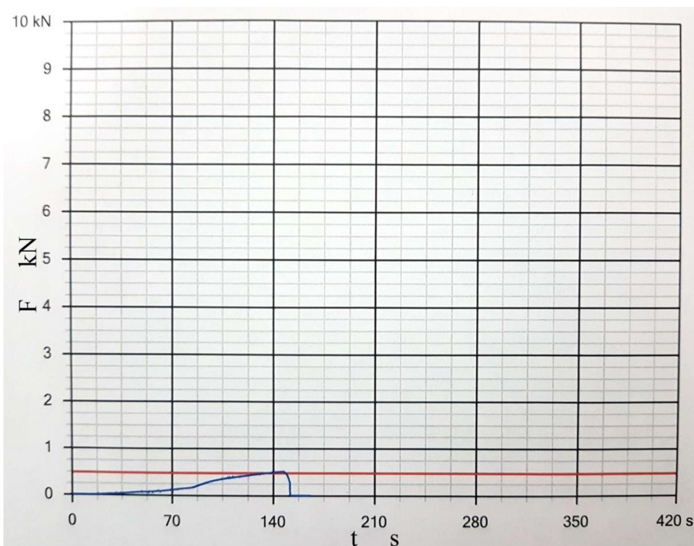
Slika 16. Dijagram sila – vrijeme za uzorak 1.6
