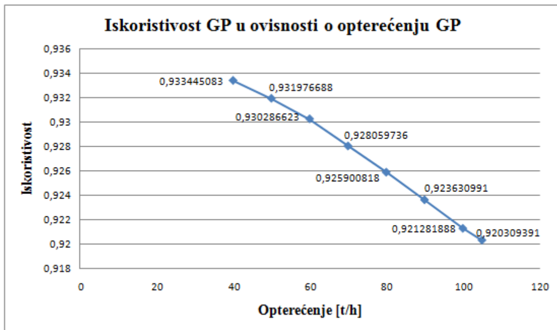
Slika 7 Ovisnost iskoristivosti generatora pare o opterećenju generatora pare
