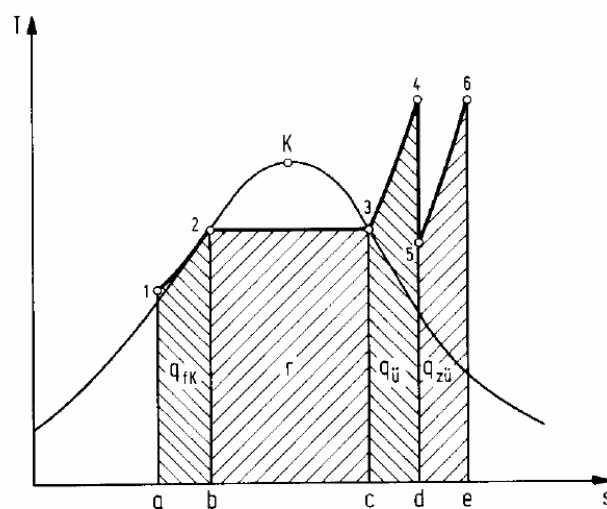
Slika 3 Proces međupregrijavanja pare
