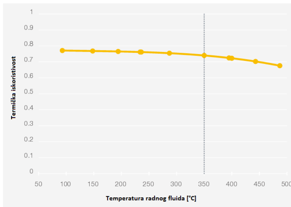
Slika 15. Termička iskoristivost paraboličkih kolektora [33]
