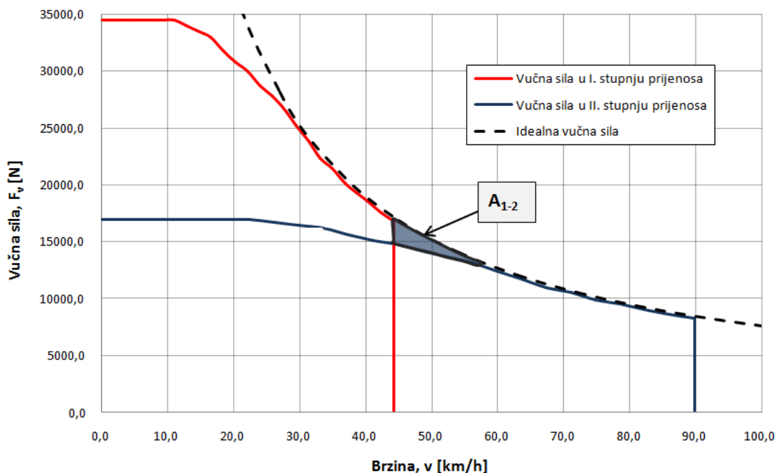
Slika 21. Vućni dijagram s ucrtanom površinom A_{1-2}
