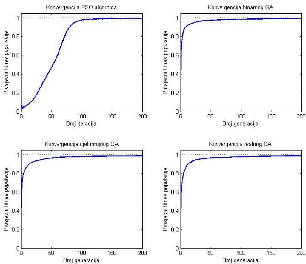
Slika 29. Konvergenije rješenja algoritama za Griewank funkciju
