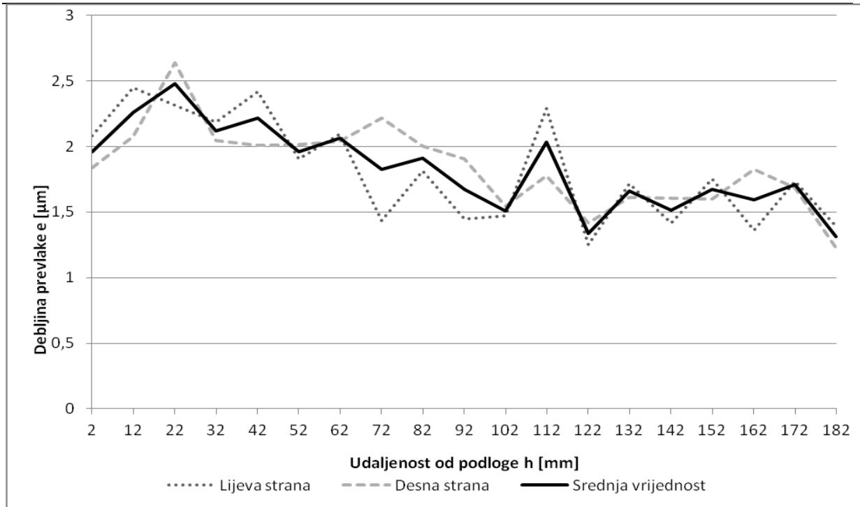
Slika 33 Ovisnost debljine TiN prevlake o udaljenosti od podloge na stražnjoj plohi ispitnog uzorka
