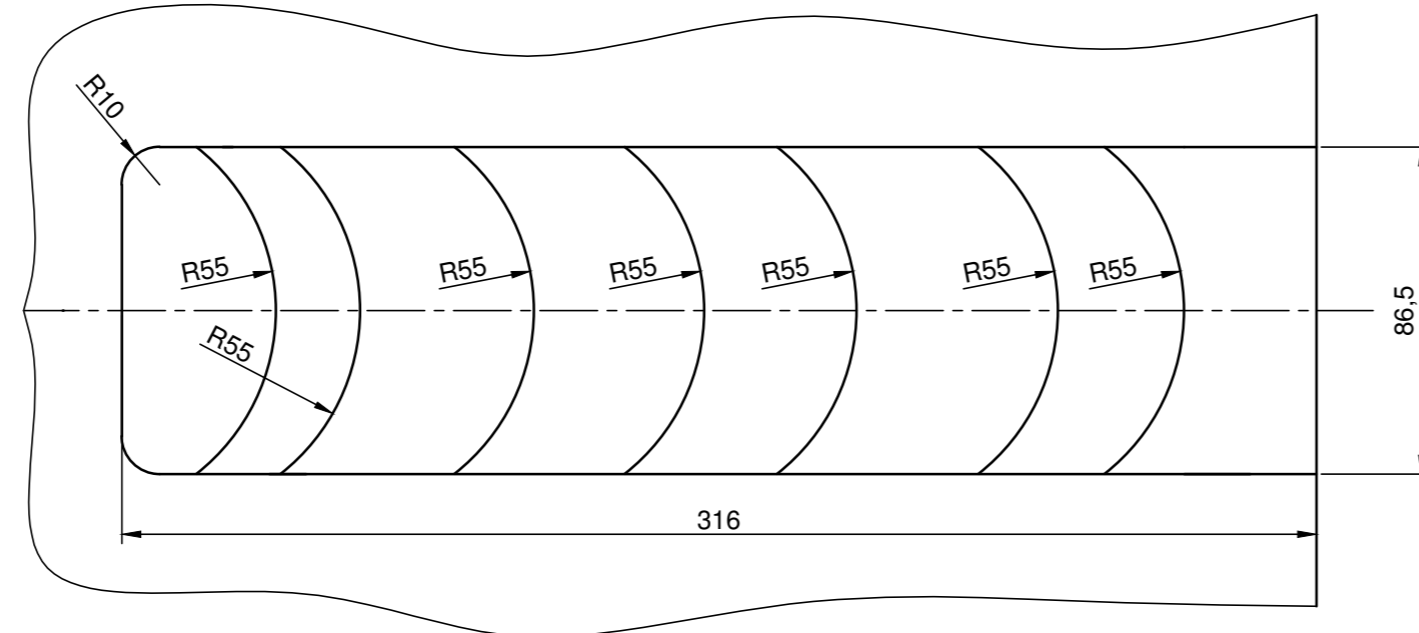
PRESJEK A-A
