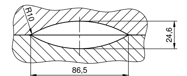
PRESJEK I - I
