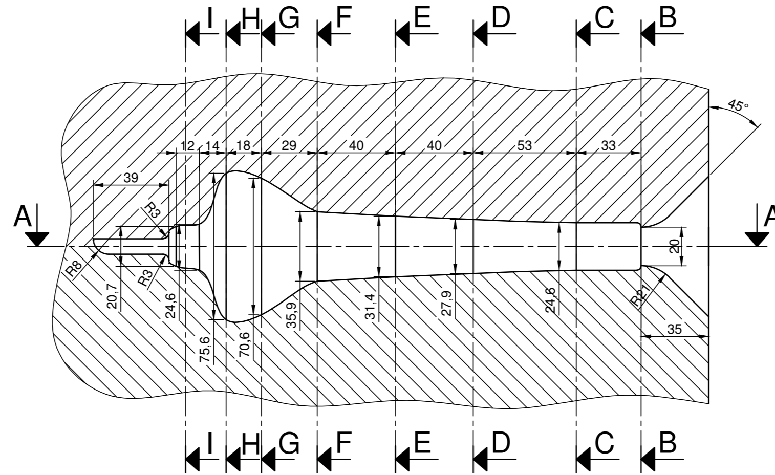
PRESJEK A-A
