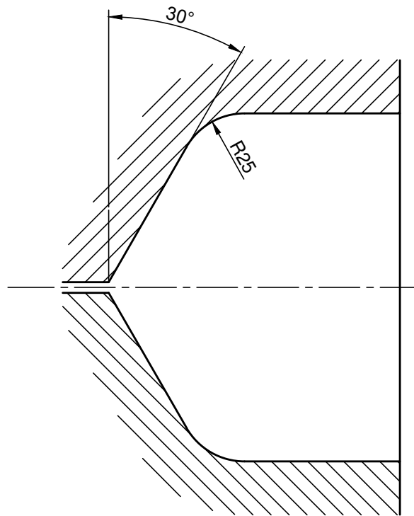
Presjek B-B
